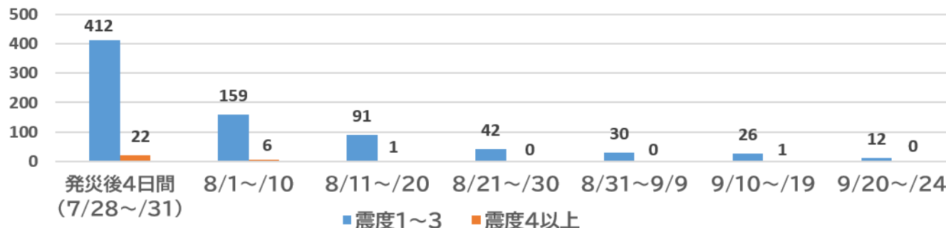
地震回数の推移
