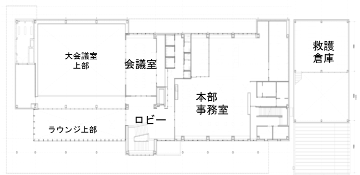
2階平面図
